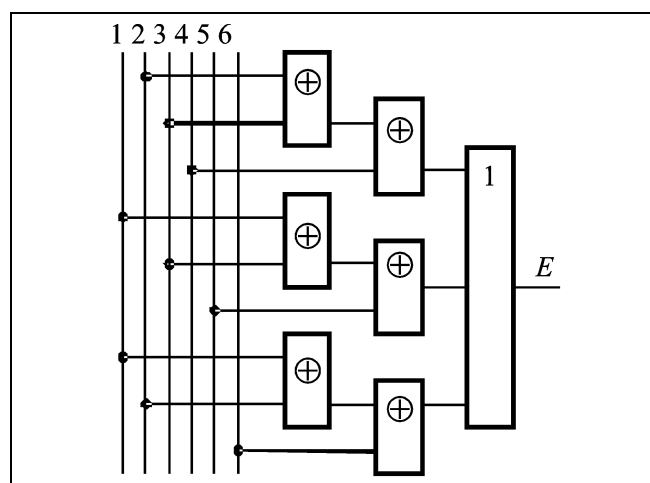
Рис. 1. Схема контроля
