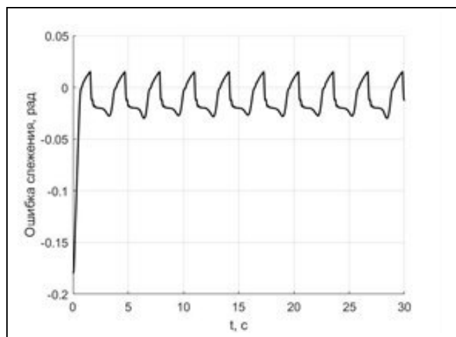
Рис. 6. График изменения ошибки e_{1a}(t) для эксперимента 2
