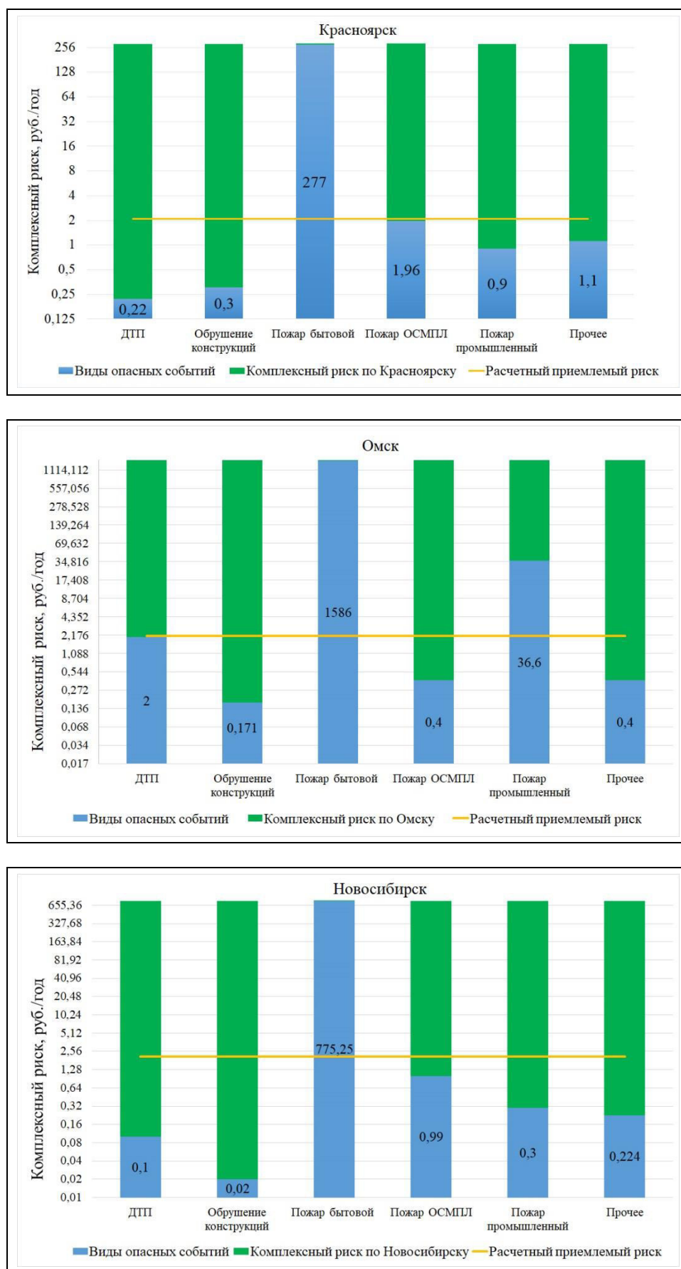
Рис. 2. Распределение значений комплексного техногенного территориального риска по видам опасностей для крупнейших городов Сибири
