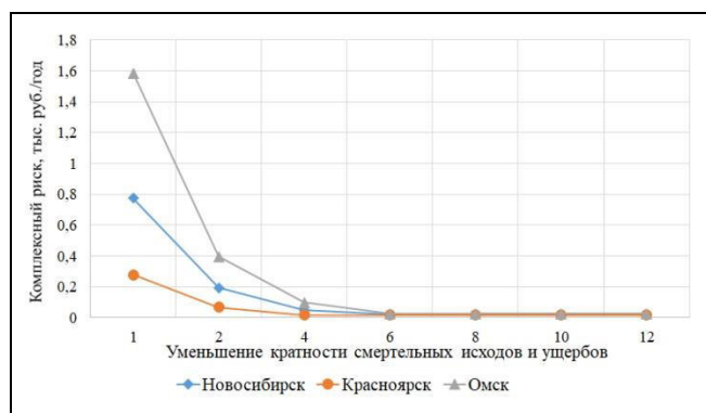
Рис. 3. Графики изменения риска при снижении размеров ущерба и смертности населения
